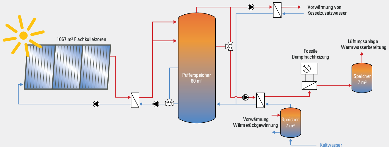
Das 1067 m 2 große Flachkollektorfeld beheizt den 60 m 3 Pufferspeicher, der wiederum Wärme für die Prozesse Kesselzusatzwasservorwärmung, Warmwasserbereitung und Lufttrocknung in der Lüftungsanlage zur Verfügung stellt.
